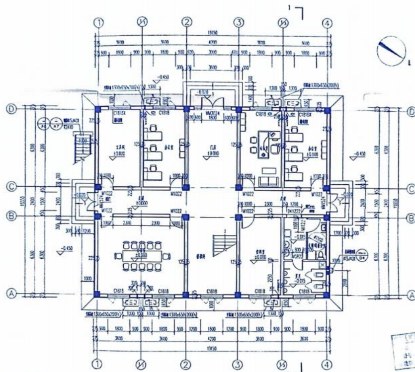
一层平面图 1:100
