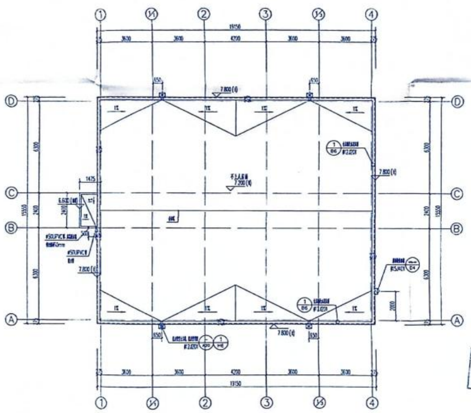
屋顶平面图 1:100
