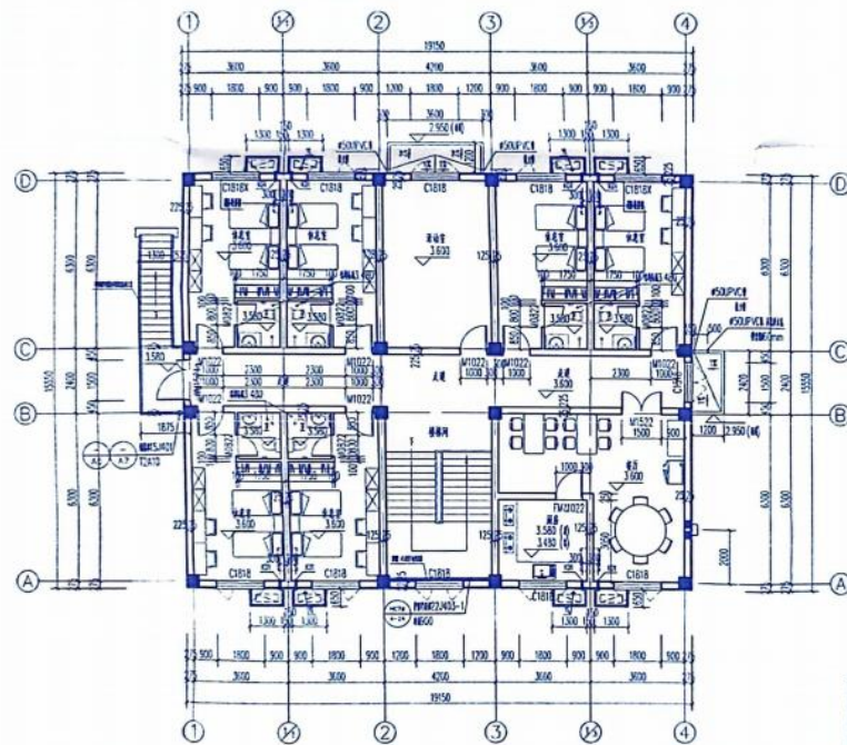
二层平面图 1:100
