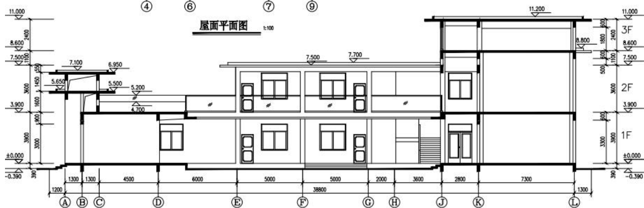
甲~甲剖面图 1:100
