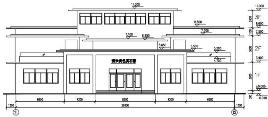
①~⑫立面图 1:100
