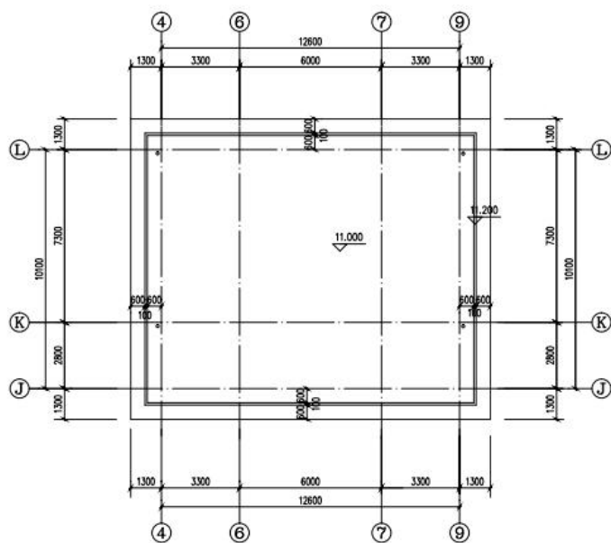
屋面平面图 1:100
