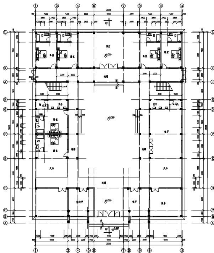
首层平面图 1:100 计容建筑面积: 1613.16 平方 不计容建筑面积: 0 平方 总建筑面积: 1613.16 平方 本层建筑面积 864.48m 2
