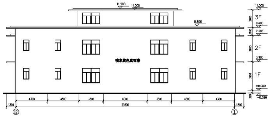
⑫~①立面图 1:100
