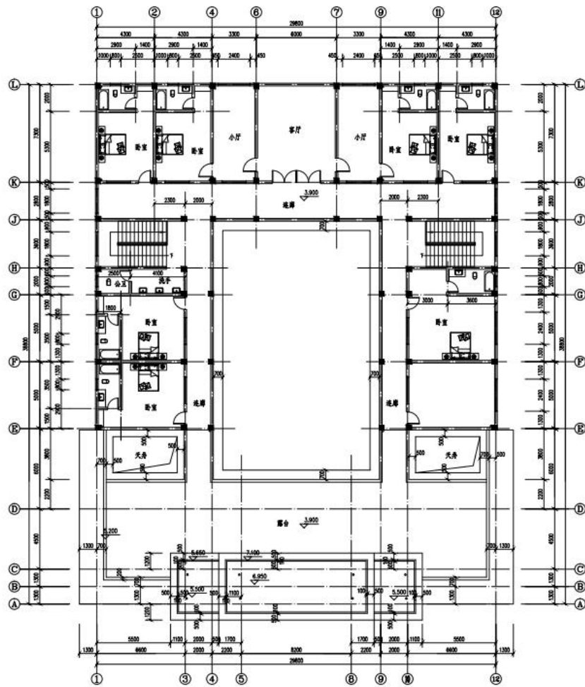
二层平面图 1:100 本层建筑面积 616.84m 2
