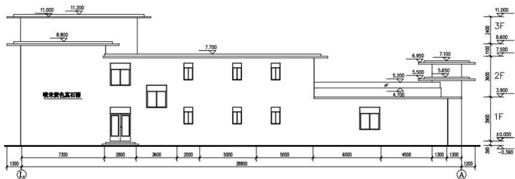
①~⑫立面图 1:100
