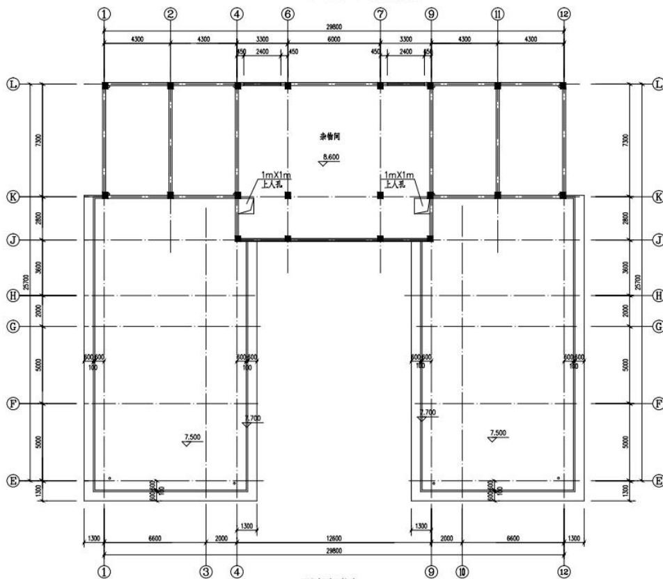
三层平面图 1:100 本层建筑面积 131.84m 2
