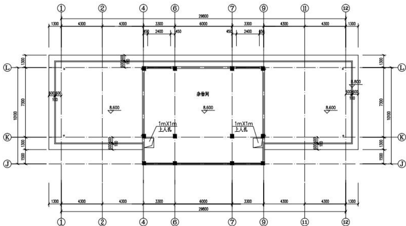
8.6米高平面图 1:100
