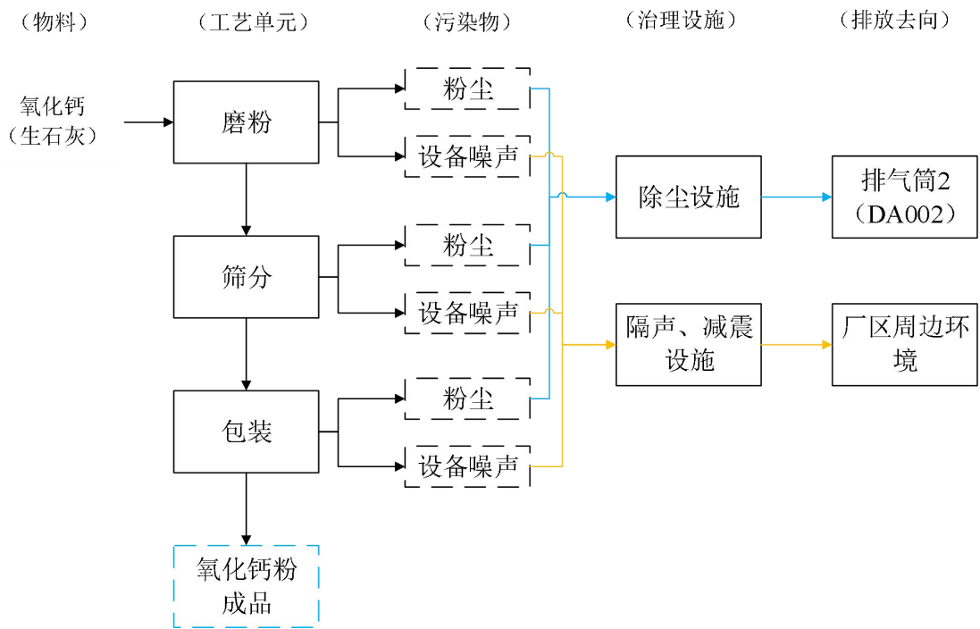
图 2-4 氧化钙工艺流程和产污环节示意图
