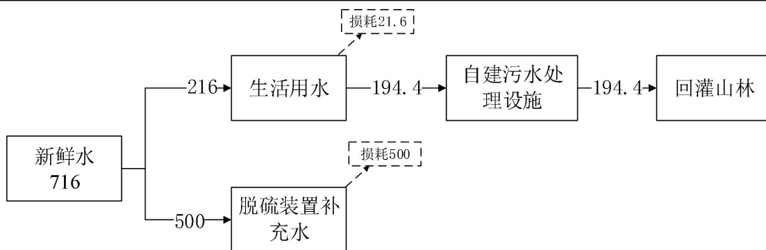
图 2-2 现有项目实际验收情况水平衡图 (t/a)
