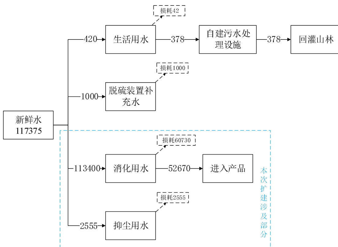
图 2-3 扩建后全厂水平衡图 (t/a)
