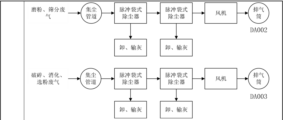
图4-1 除尘系统工艺流程
