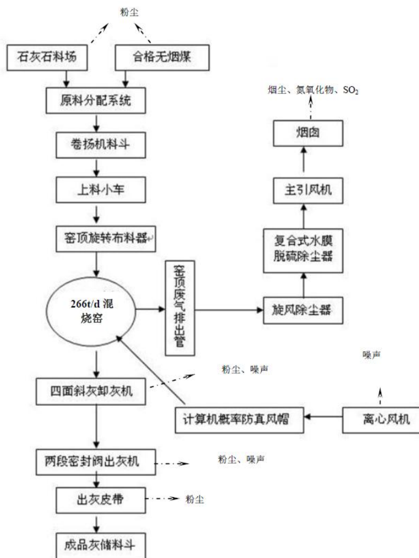
图 2-6 现有项目石灰生产工艺流程图
