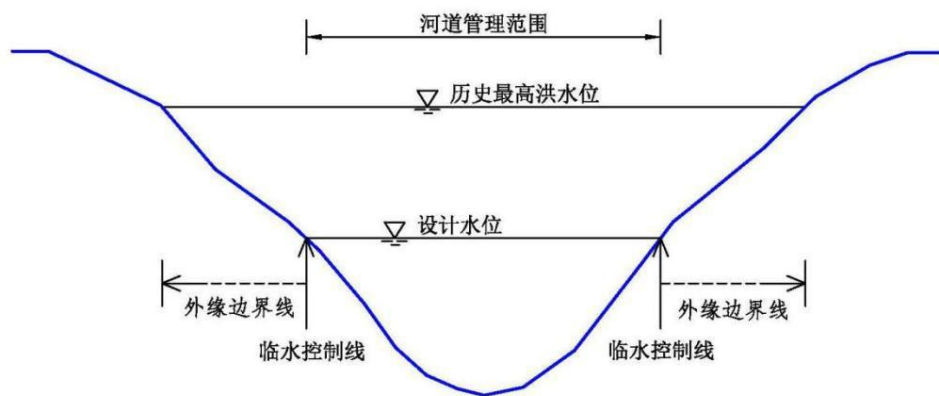
图7-1-3 无堤防山丘区河道岸线控制线示意图
