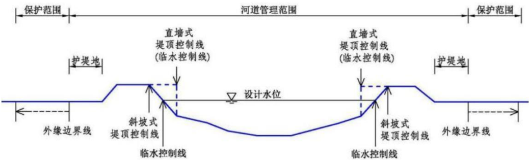
图7-1-1 有堤防河道岸线控制线示意图
