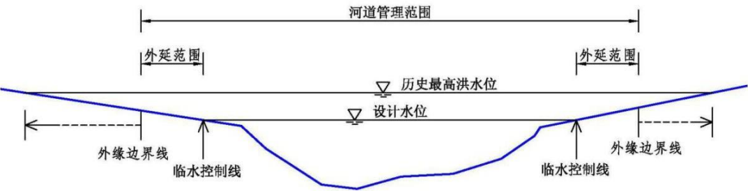
图7-1-2 无堤防平原区河道岸线控制线示意图
